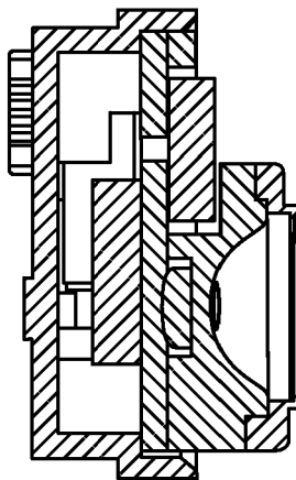
Section A-A FIG. 90C
