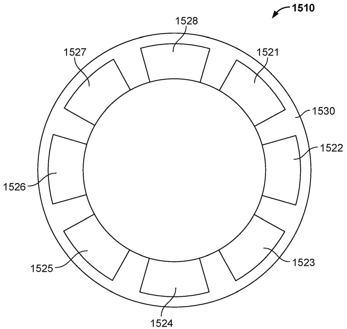
FIG. 14A
