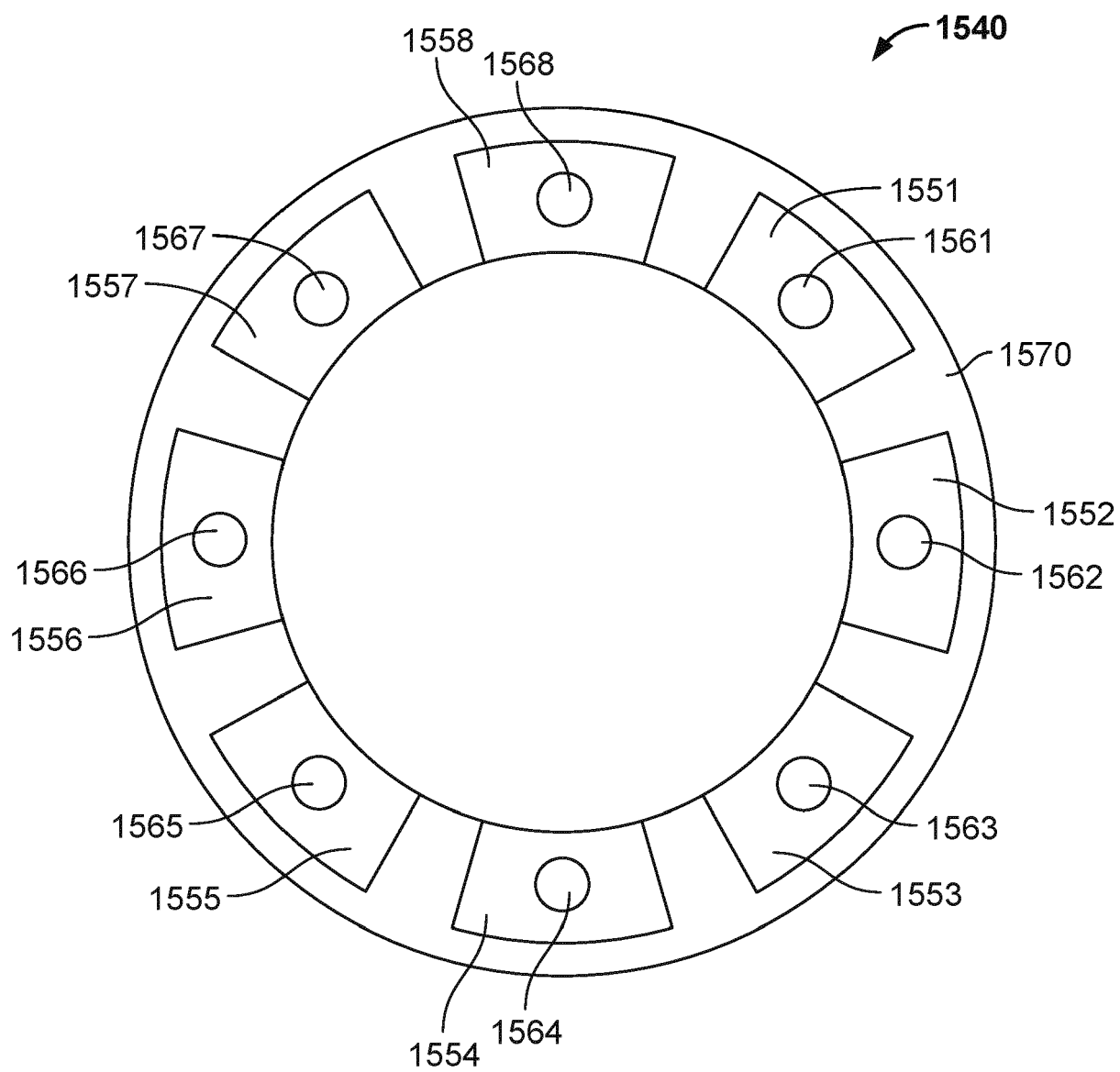
FIG. 14B
