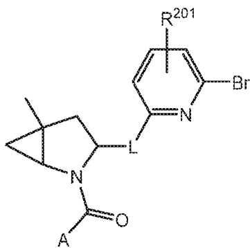
Formula II-40
