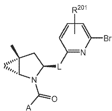
Formula II-42
