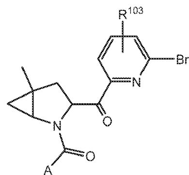
Formula III-46
