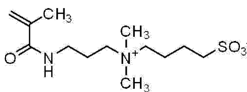
Monomer M-2
