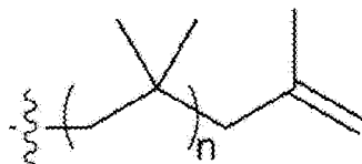
[Formula b-1]
