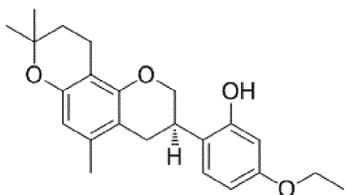
<Compound 9a>
