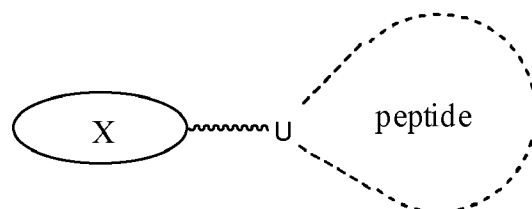
Formula 3-I-A
