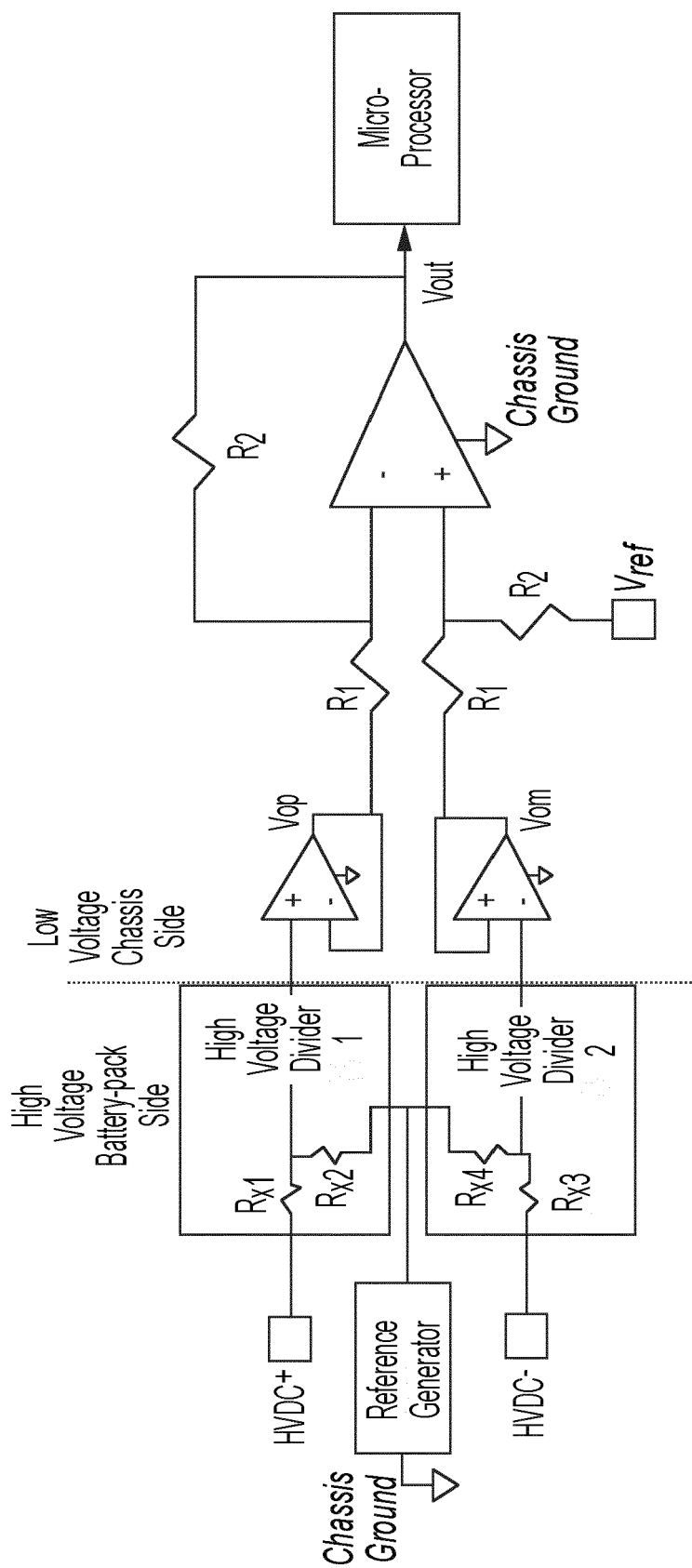
FIG. 3A PRIORART
