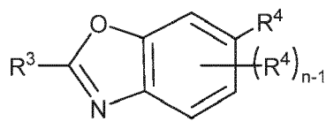
(IIIf),
