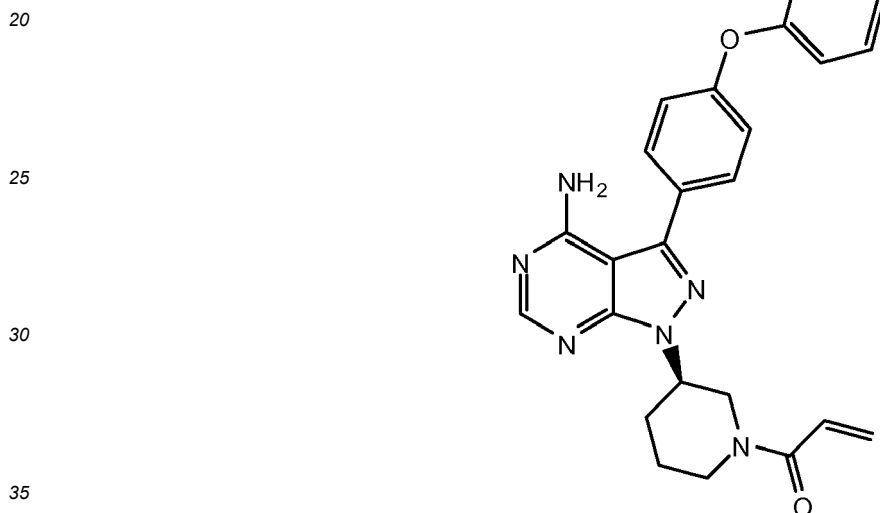
Ibrutinib.
