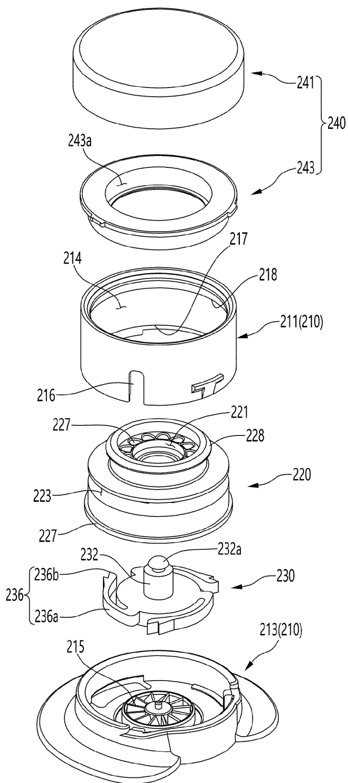
FIG. 12
