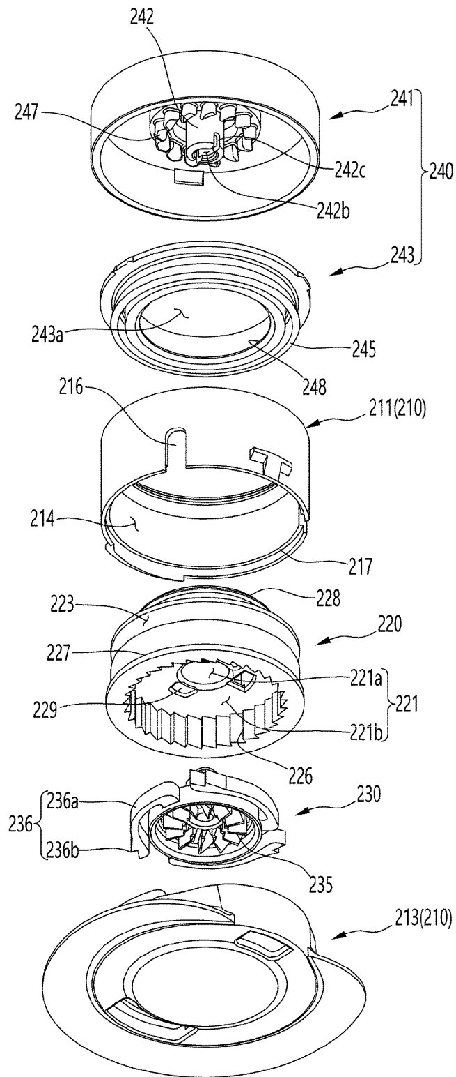
FIG. 13
