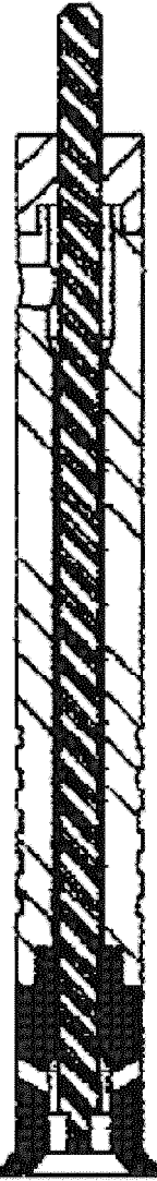
FIG. 9H
