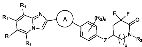
Formula (IIa);
