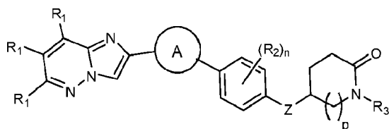
Formula (Ie);
