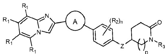
Formula (Ia);
