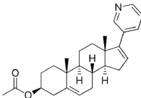
Abiraterone Acetate
