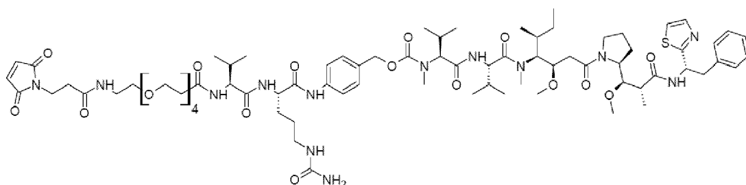
vc-MMAE:
