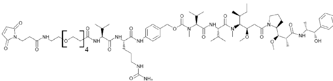
vc-MMAE:
