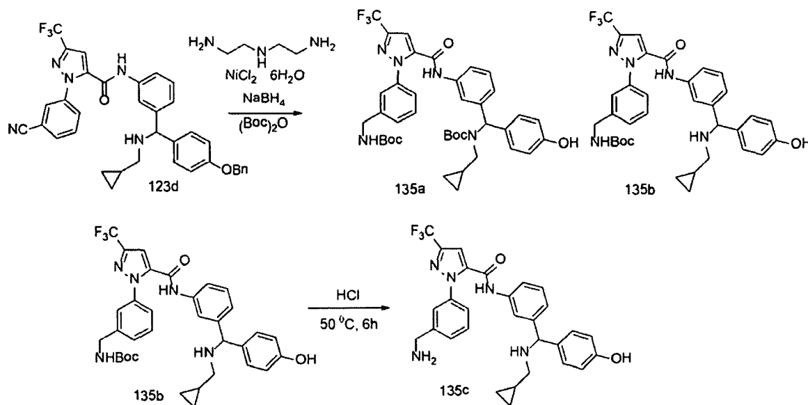
Scheme 135
