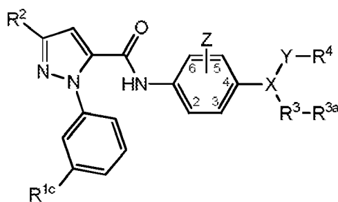
(XIV).
