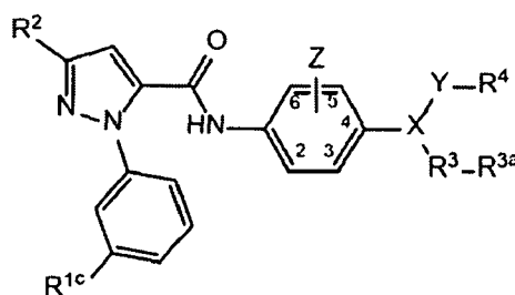
(XV)
