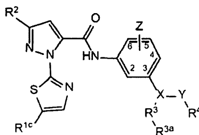
(XII).
