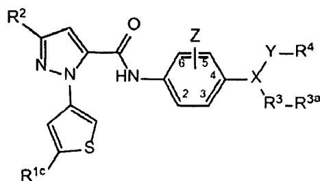
(XXII).
