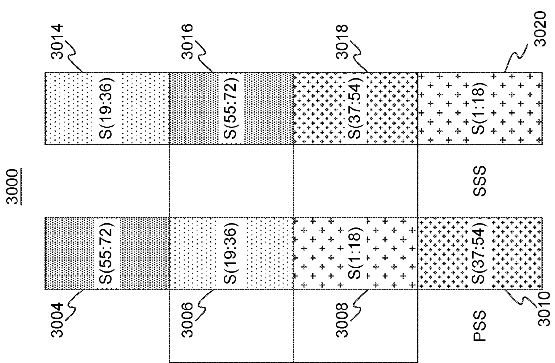
3002 PBCH1 PBCH2 3012 FIG. 30
