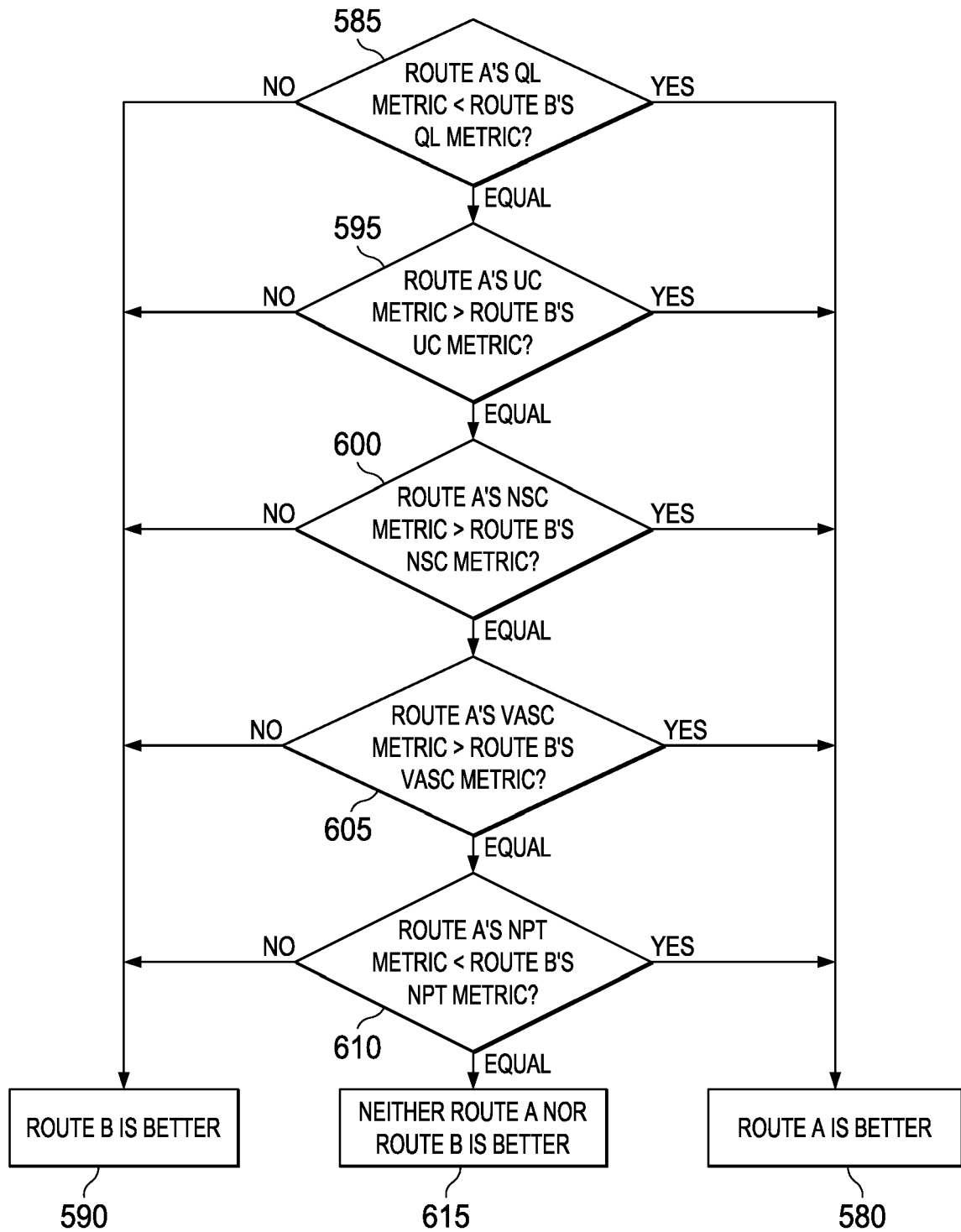
FIG. 13B
