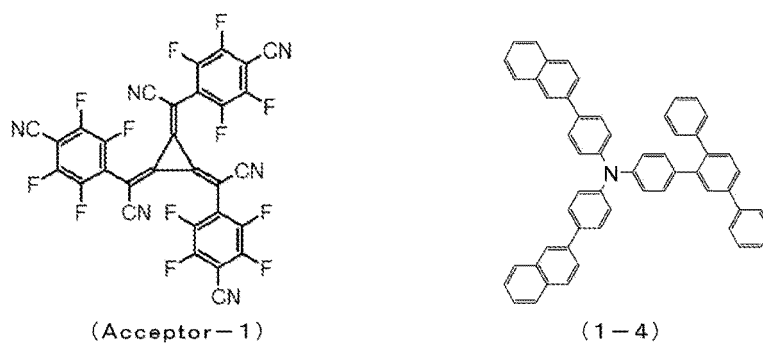
[Chem. 23]
