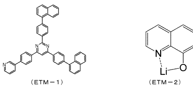
[Chem. 25]
