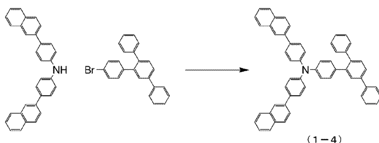
[Chem. 6]
