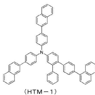
[Chem. 23]
