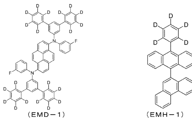
[Chem. 25]
