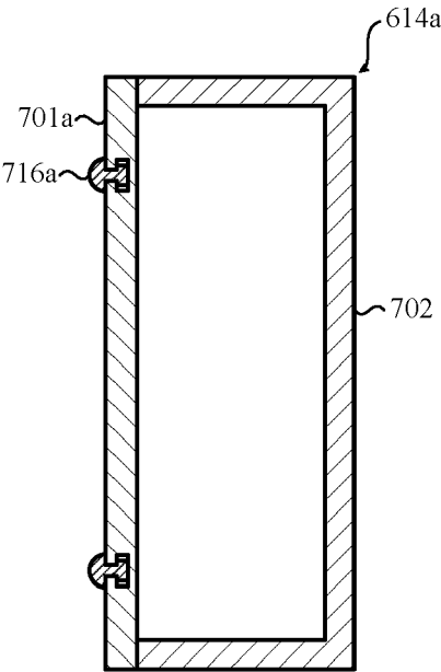
SECTION B-B FIG. 7A
