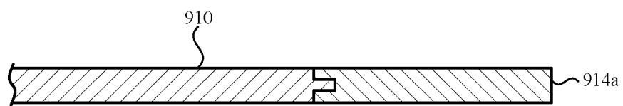
SECTION D-D FIG. 9B
