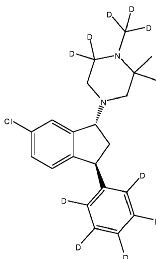
(1R,3S)-(V),
