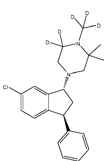
(1R,3S)-(V),
