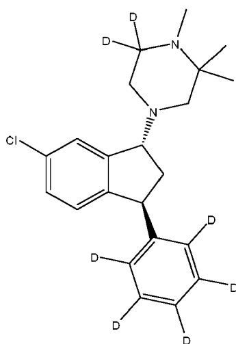
(1R,3S)-(VII).
