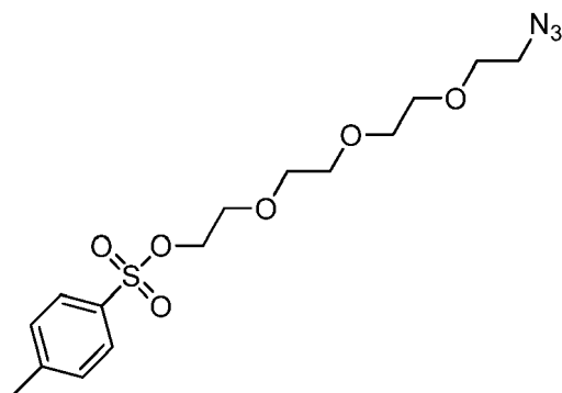
2-(2-(2-(2-azidoethoxy)ethoxy)ethoxy)ethyl 4-methylbenzenesulfonate
