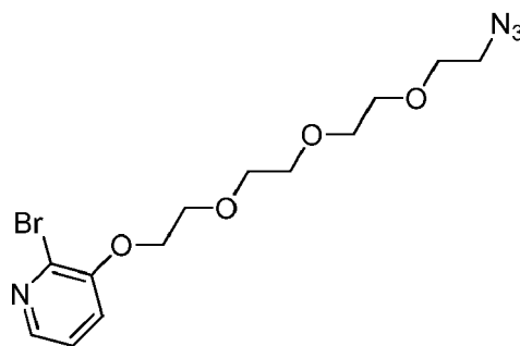
3-(2-(2-(2-(2-azidoethoxy)ethoxy)ethoxy)ethoxy)-2-bromopyridine
