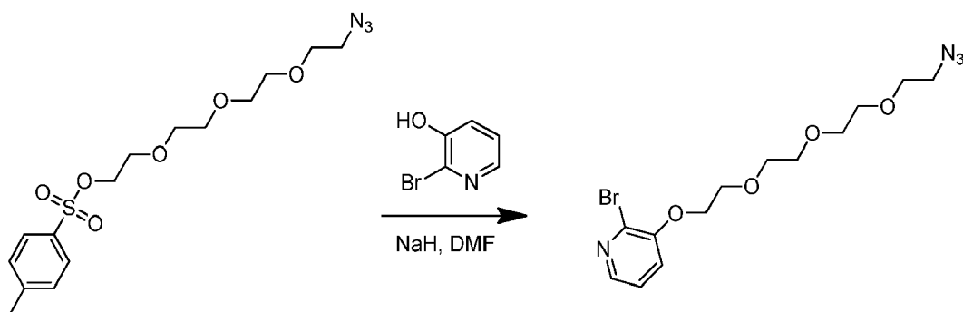
3-(2-(2-(2-(2-azidoethoxy)ethoxy)ethoxy)ethoxy)-2-bromopyridine
