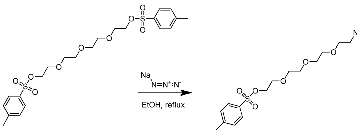
2-(2-(2-(2-azidoethoxy)ethoxy)ethoxy)ethyl 4-methylbenzenesulfonate
