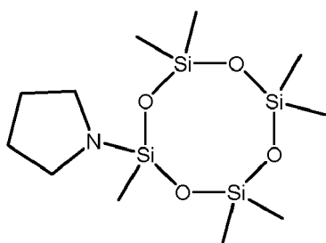
2-pyrrolidino-2,4,4,6,6,8,8-heptamethylcyclotetrasiloxane
