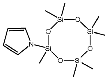
2-pyrrolyl-2,4,4,6,6,8,8-heptamethylcyclotetrasiloxane
