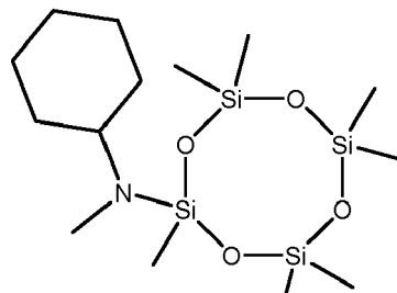
2-cyclohexylmethylamino-2,4,4,6,6,8,8-heptamethylcyclotetrasiloxane
