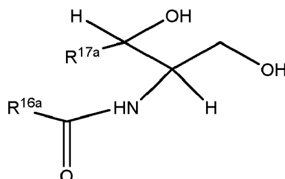
(IXa)
