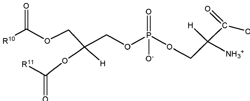
(VI)
