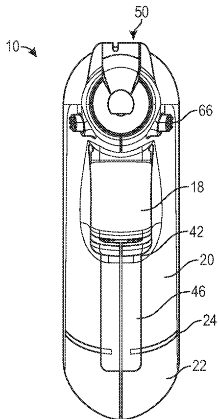
FIG. 2B
