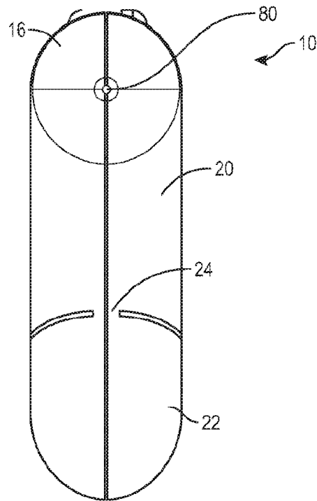
FIG. 2C
