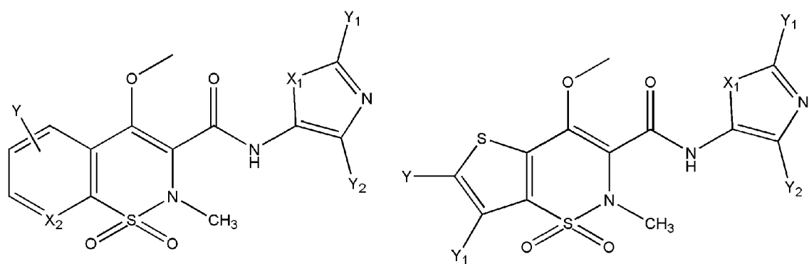
[Chem.35]
