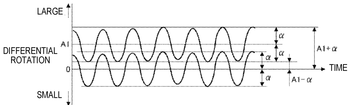
[FIG. 8A]
