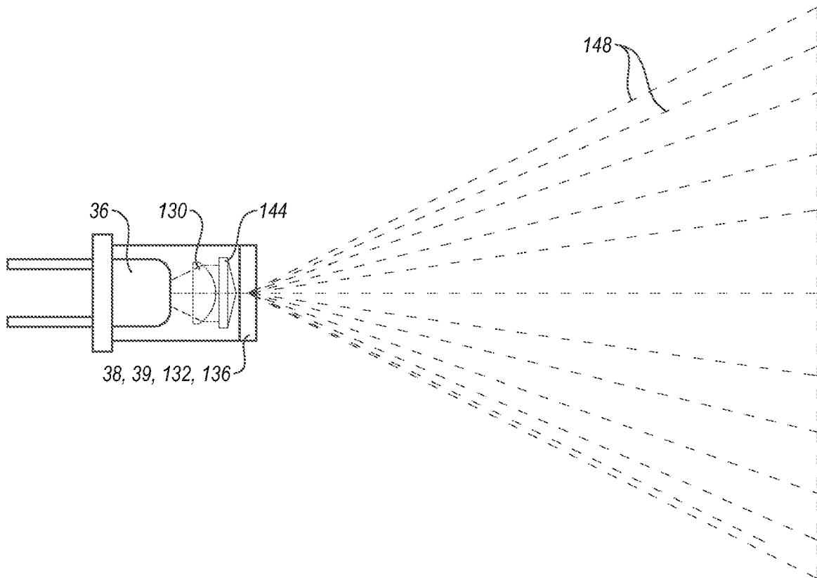
FIG. 23B
