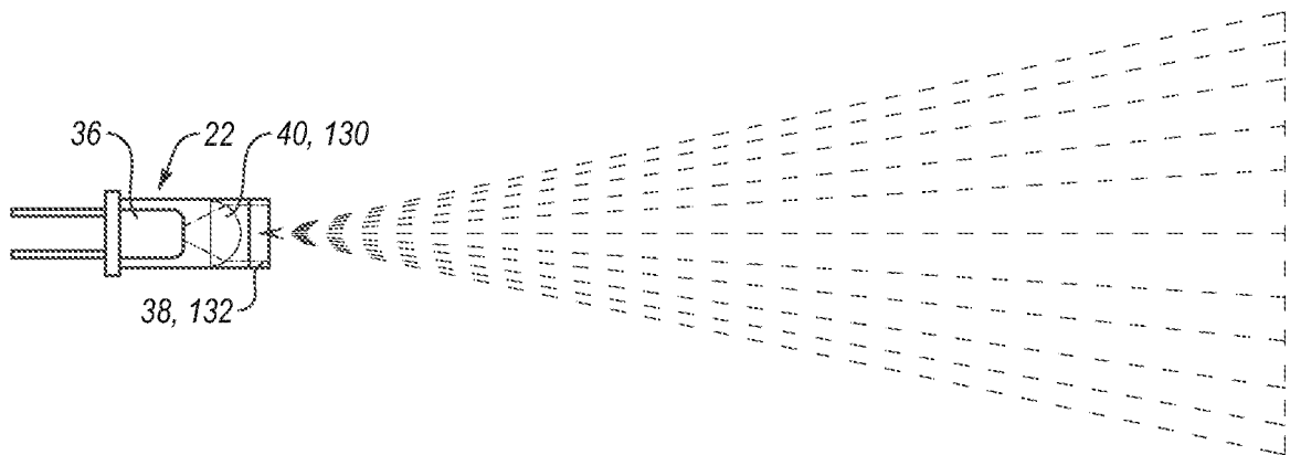
FIG. 20A
