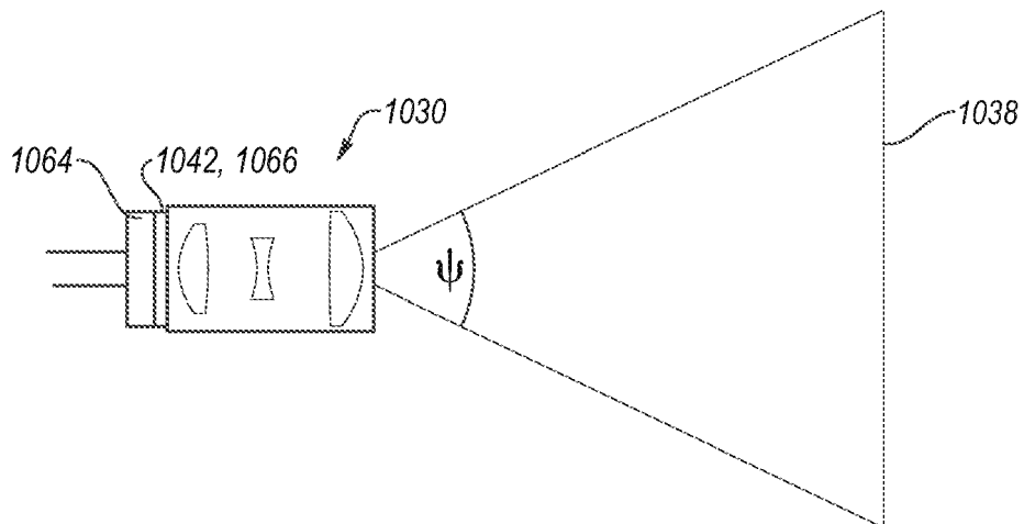
FIG. 29B
