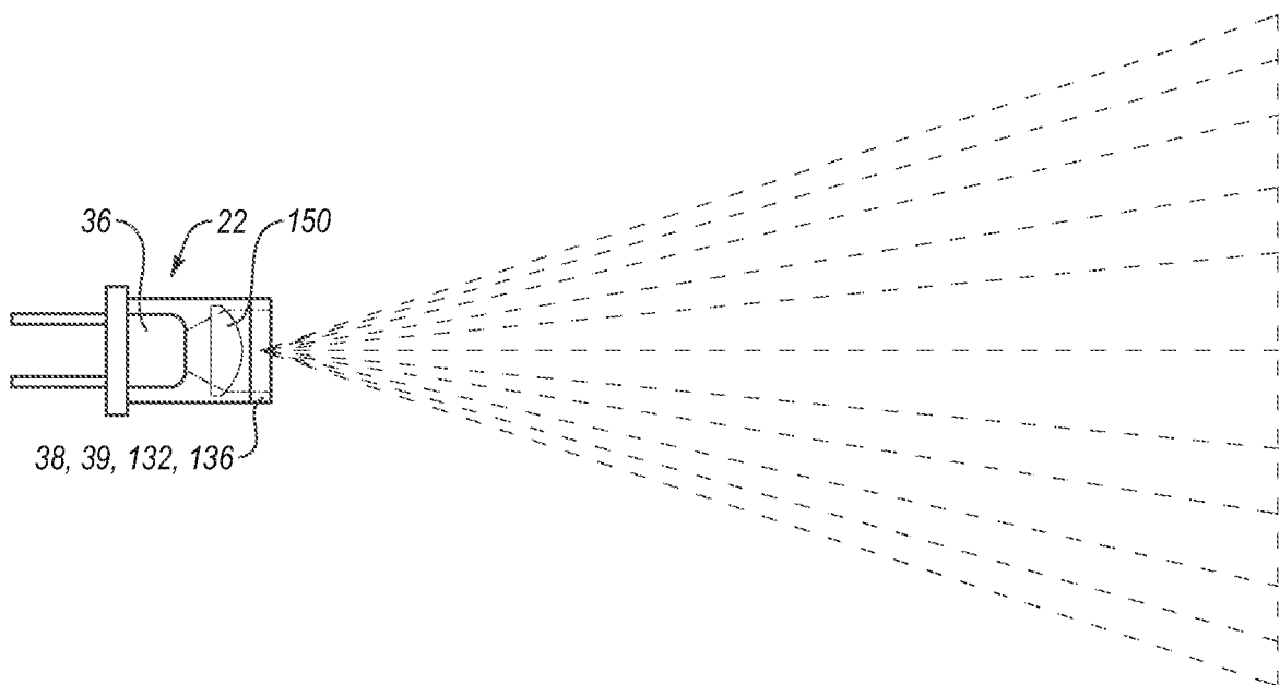
FIG. 24B
