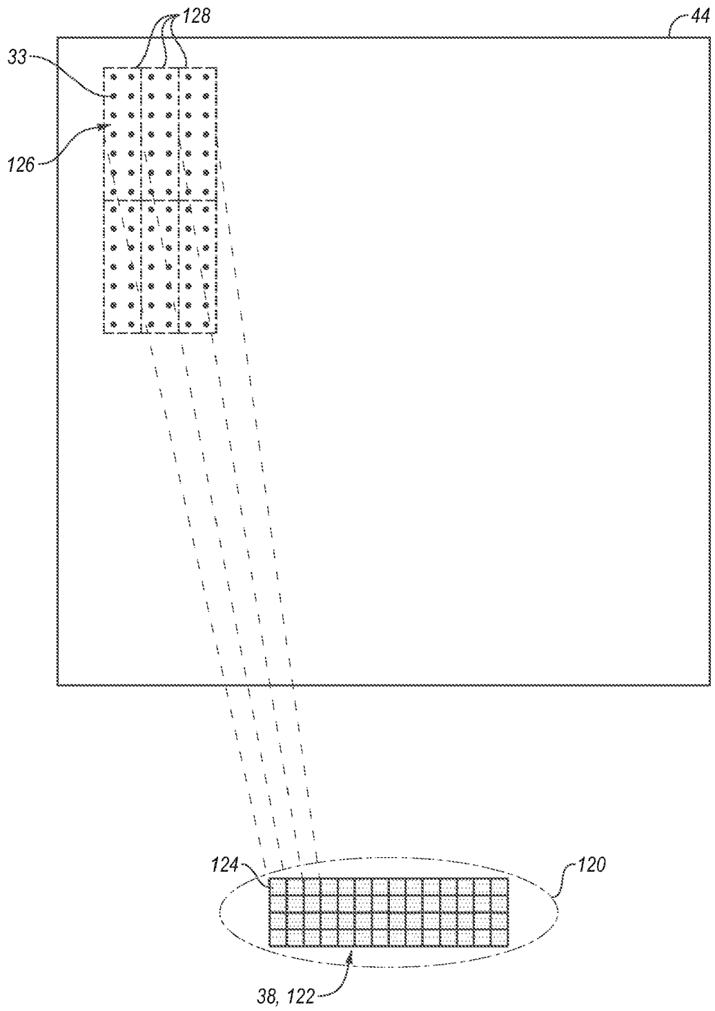
FIG. 19B
