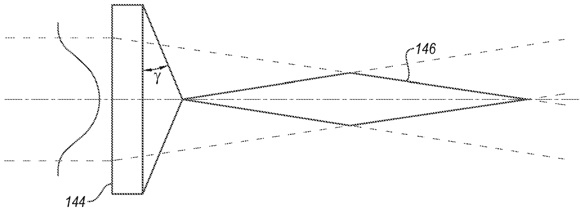
FIG. 23A
