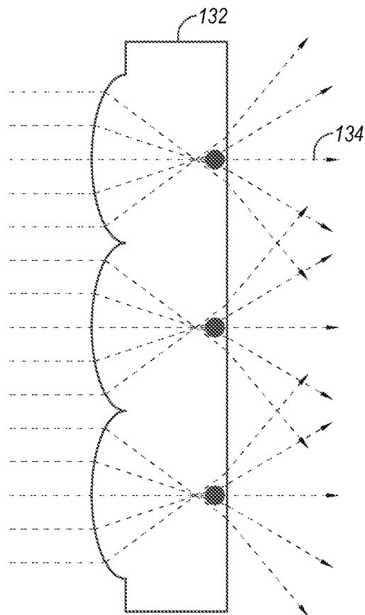
FIG. 20B
