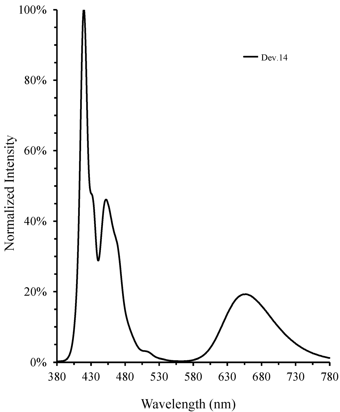
FIG. 22
