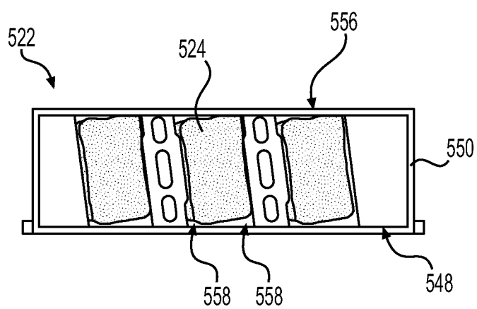
FIG. 25B
