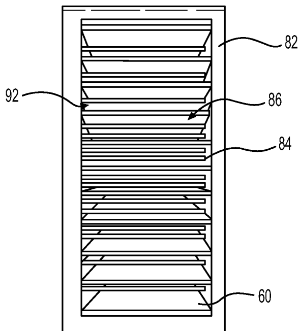
FIG. 6C
