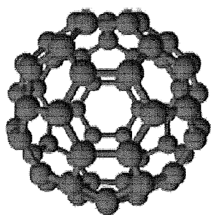
Fullerene
