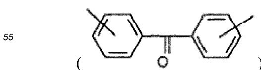
di-benzophenone
