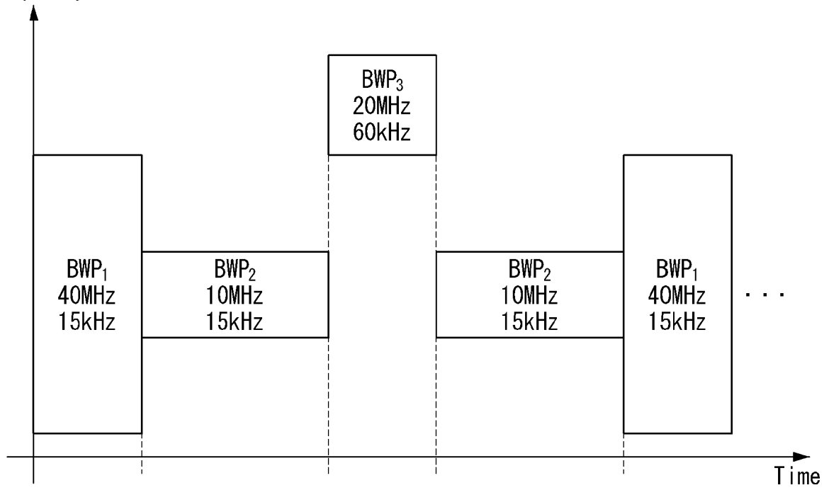
【FIG. 8】 Frequency
