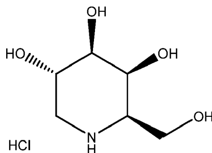
Migalastat HCl
