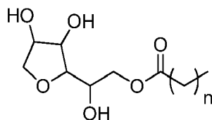
Sorbitan Ester n = 6-12
