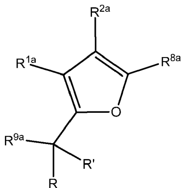
Formula Va
