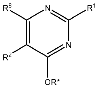
Formula VIIt
