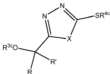
Formula Ic
