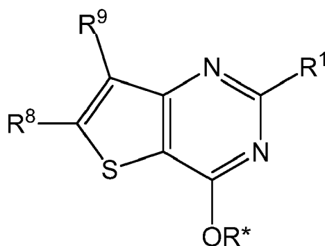
Formula VIIt1
