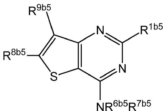
Formula VIIIb5
