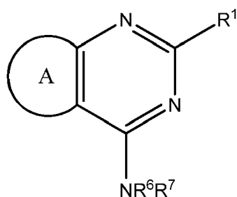
Formula VIIb
