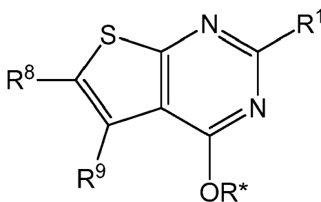
Formula VIIt2
