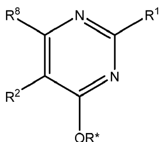
Formula VIIt
