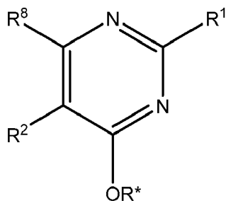
Formula VIIt
