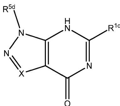
Formula VIId
