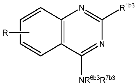
Formula VIIIb3
