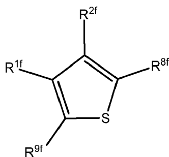
Formula Vf
