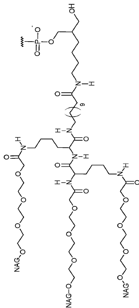
(NAG13)
