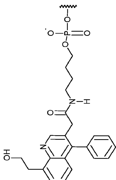
(PAZ)
