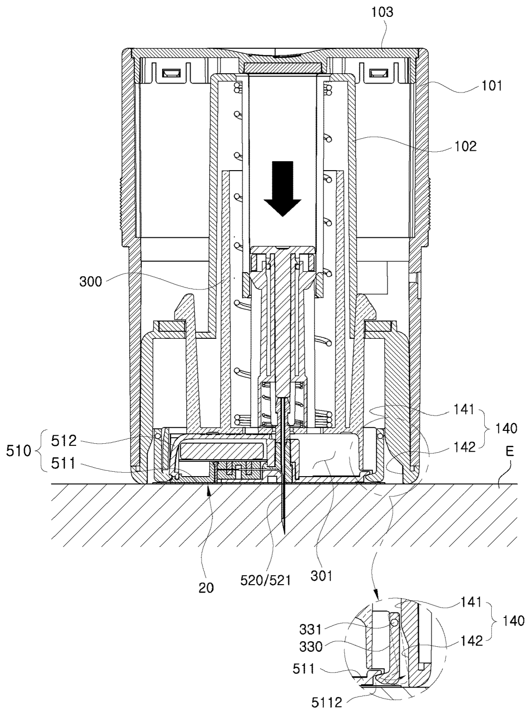
FIG. 18B
