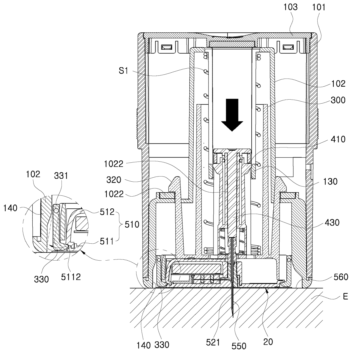
FIG. 22A
