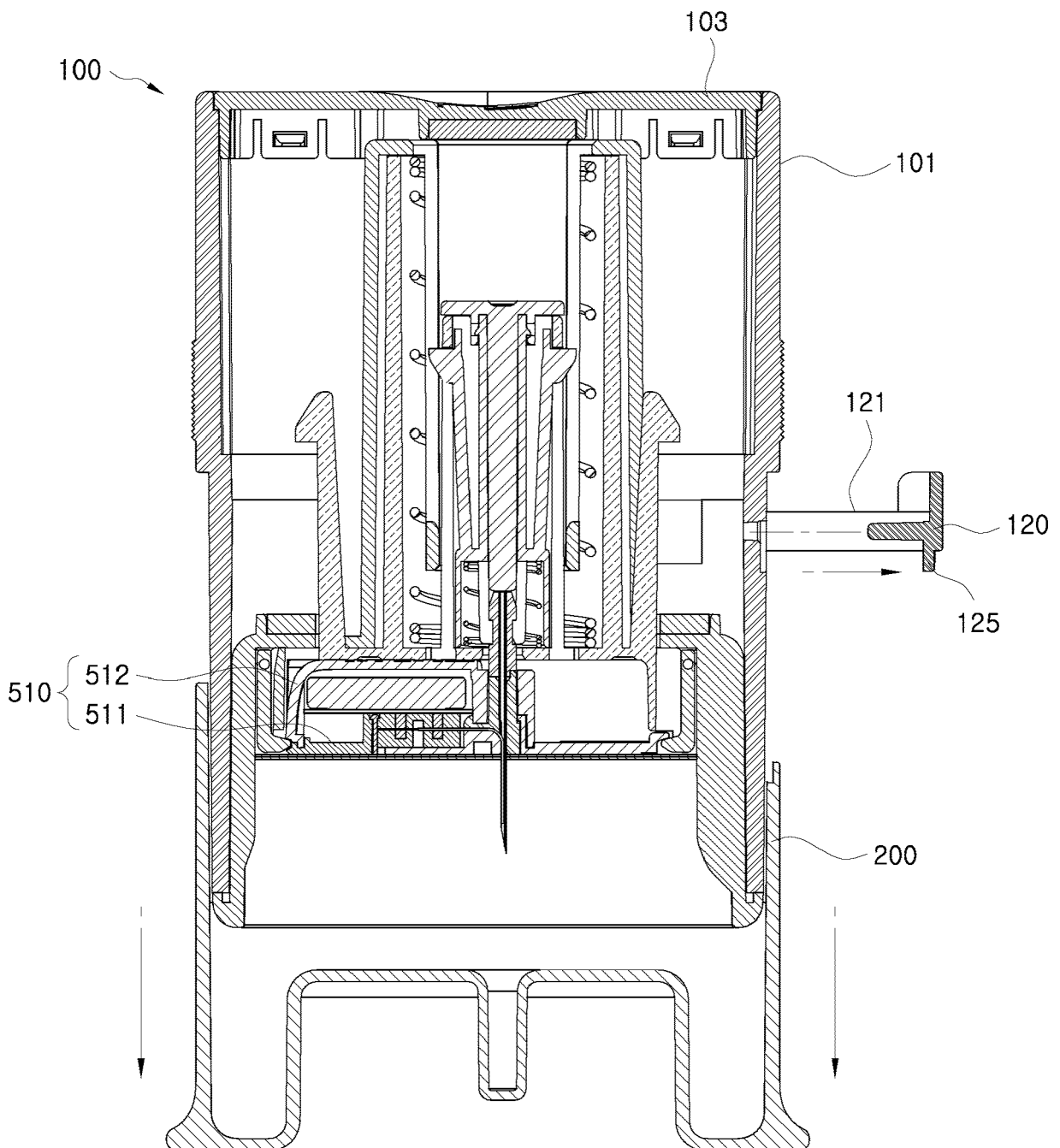
FIG. 16B
