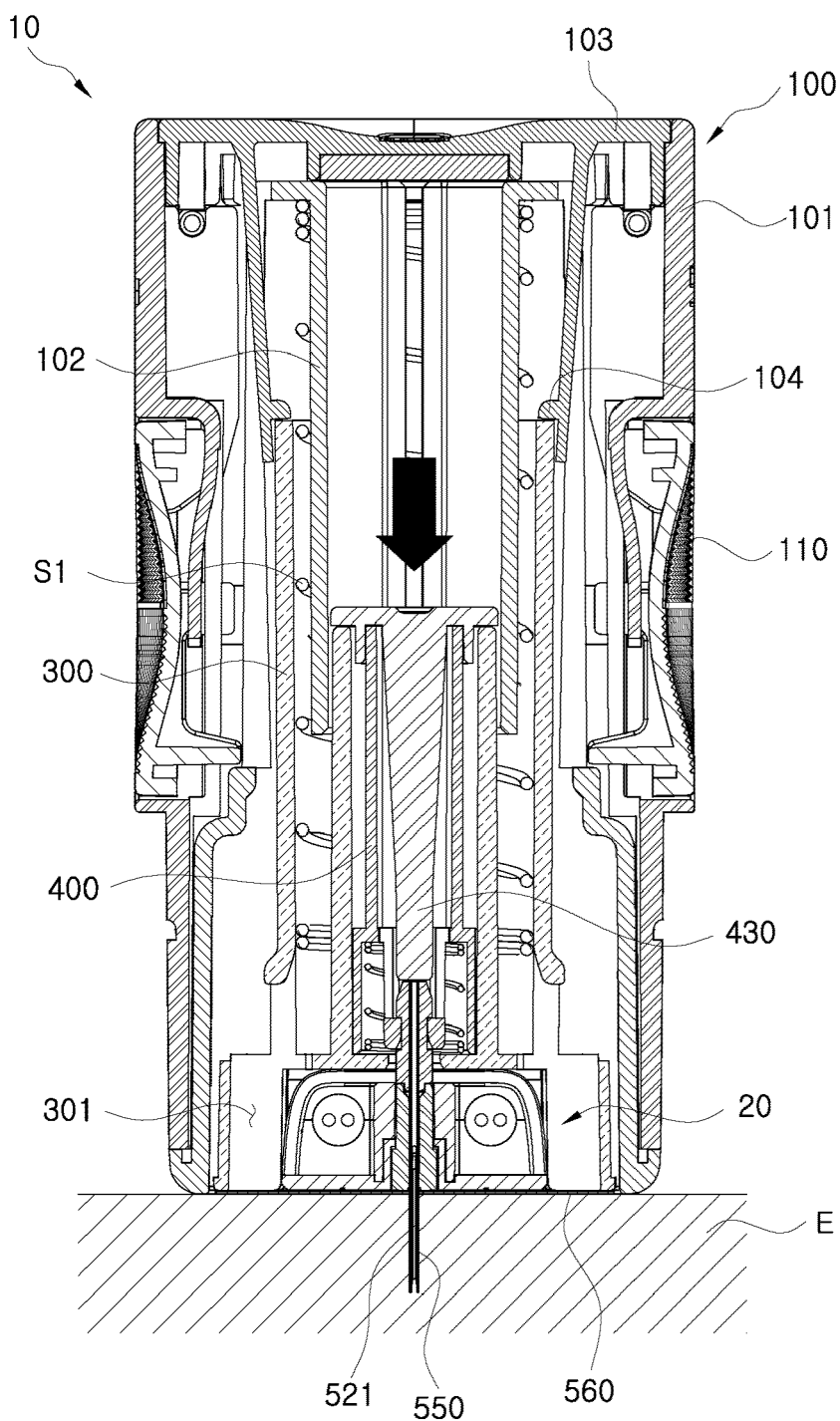
FIG. 22B
