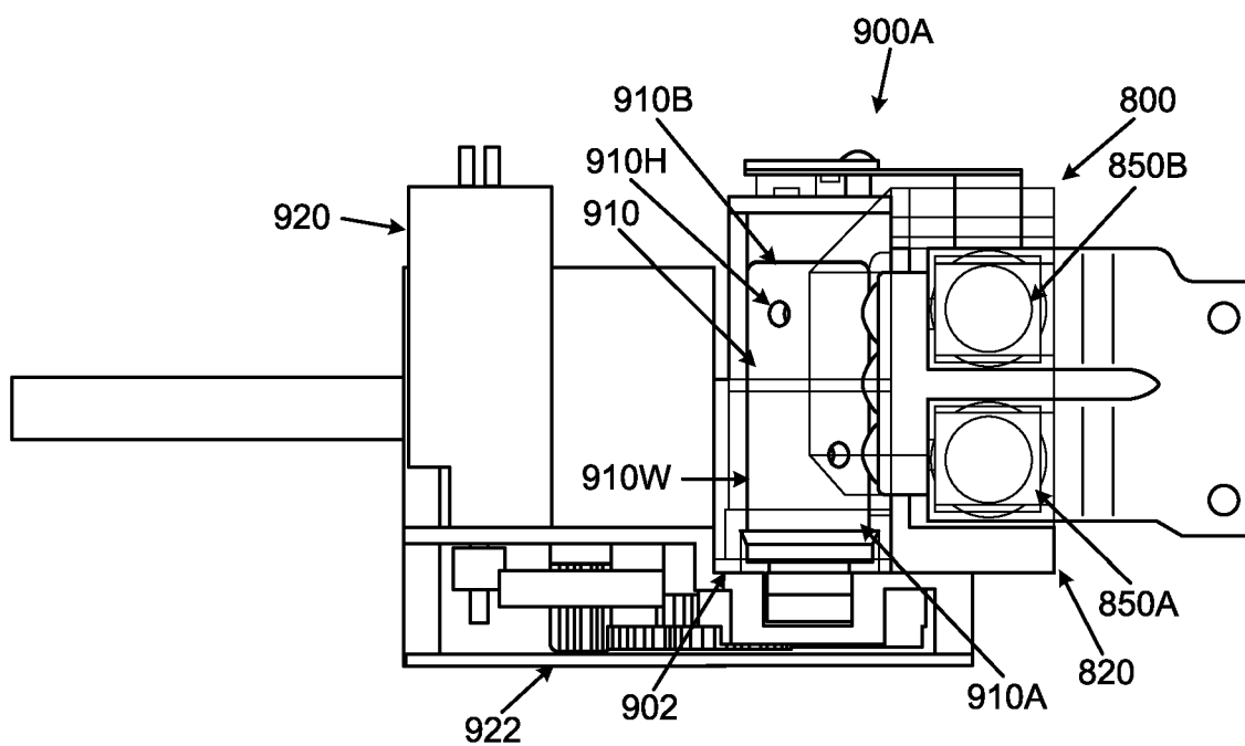
FIG. 27B
