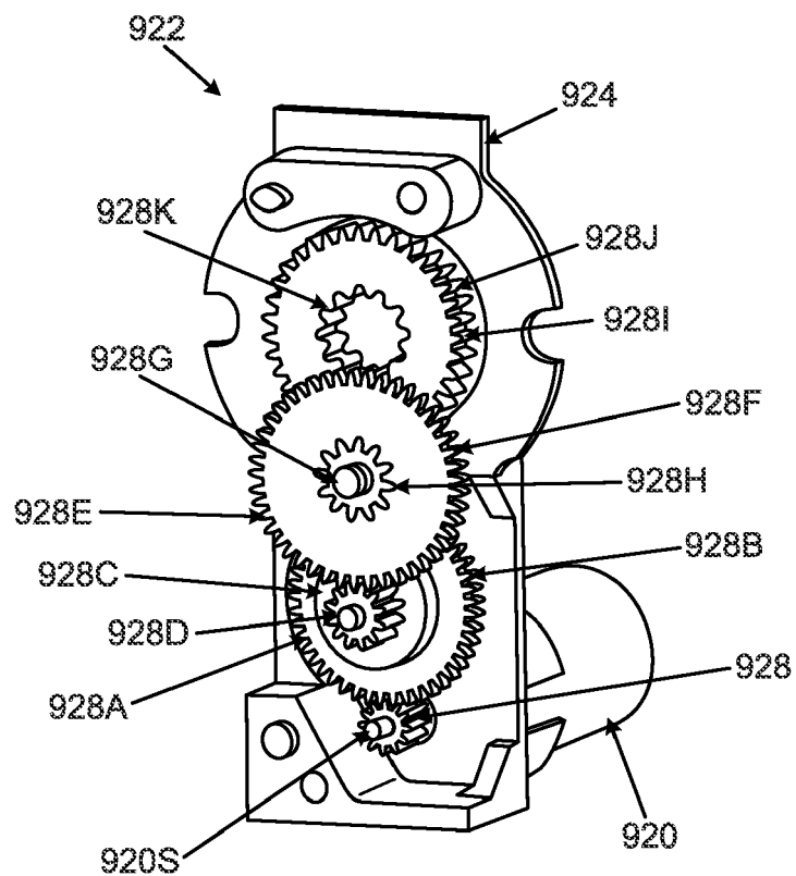
FIG. 40C
