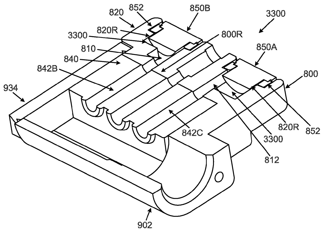
FIG. 33F
