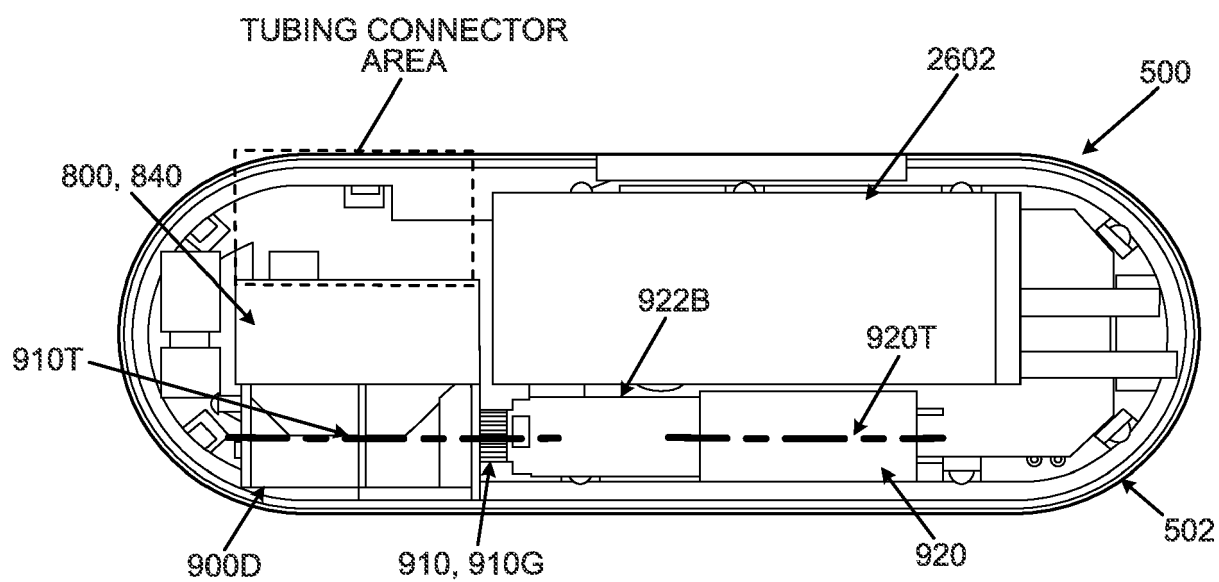
FIG. 41A
