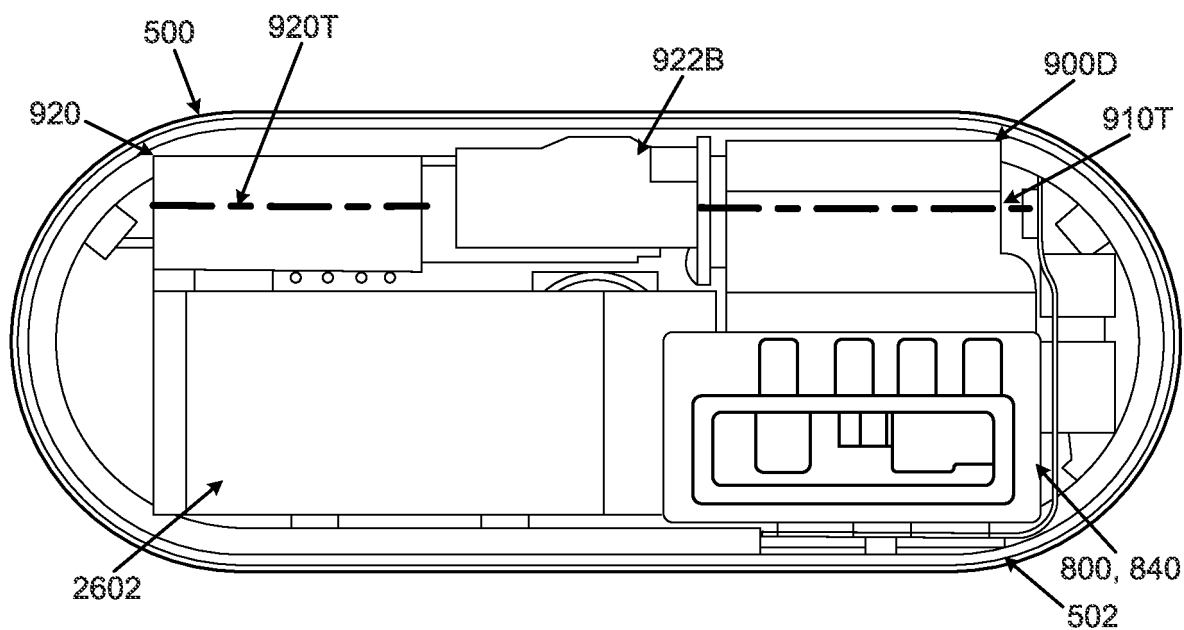
FIG. 41B
