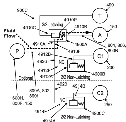
FIG. 49A
