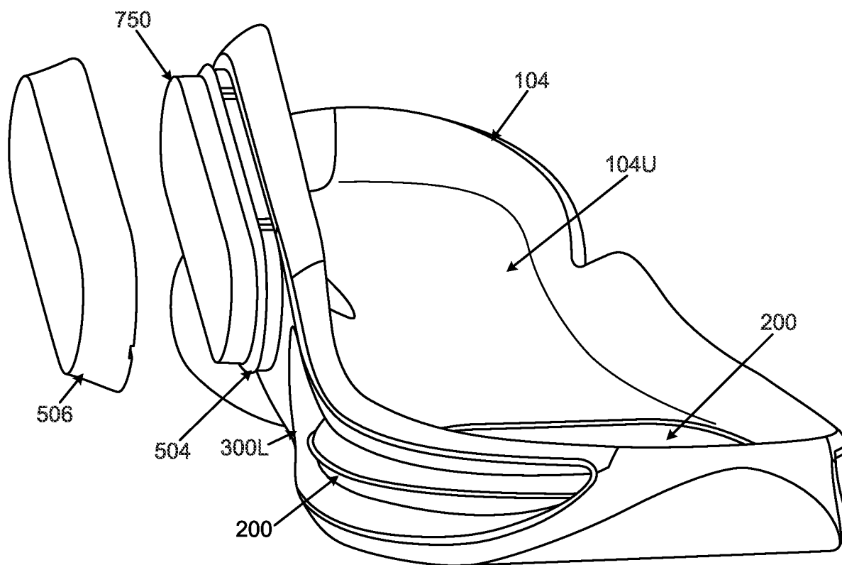
FIG. 15F
