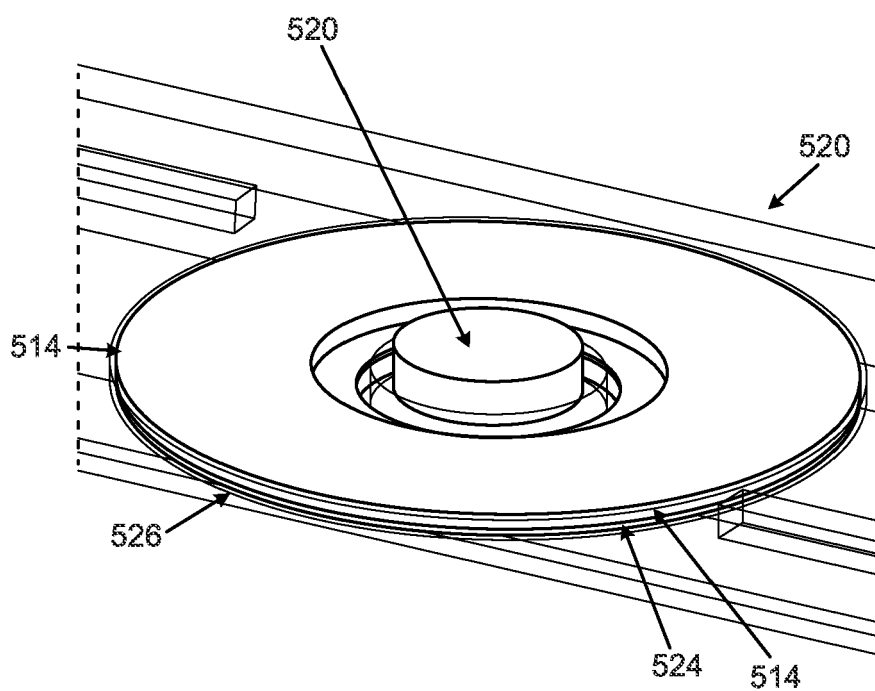
FIG. 18A
