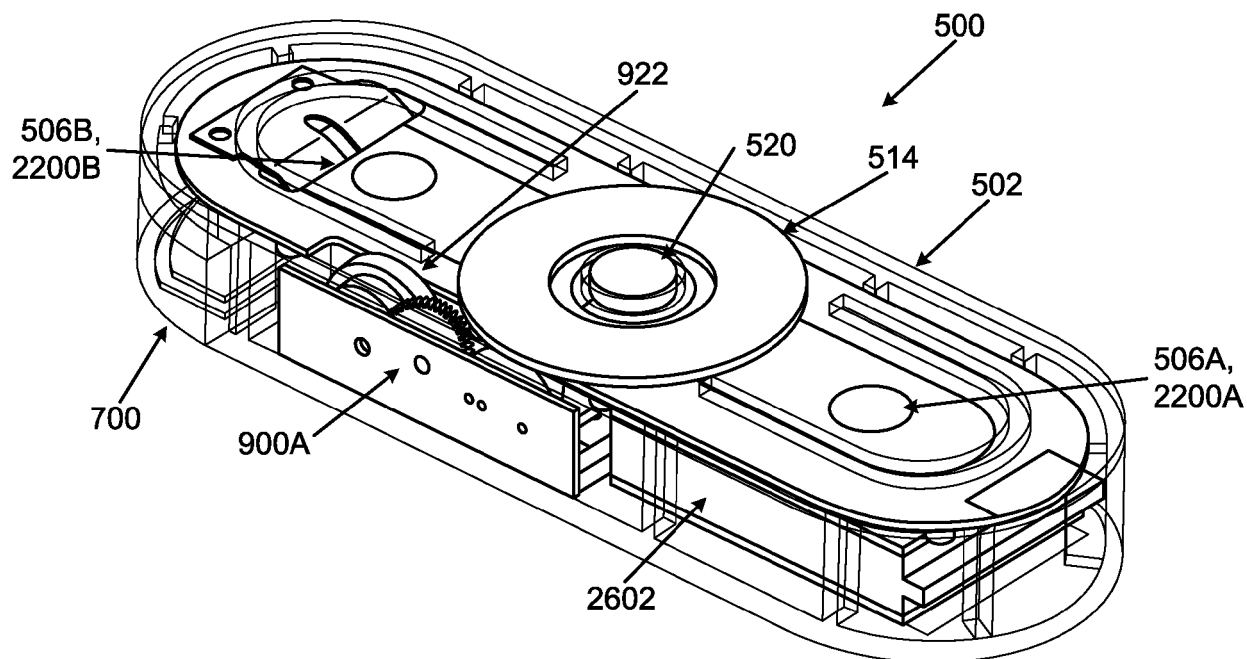
FIG. 26A
