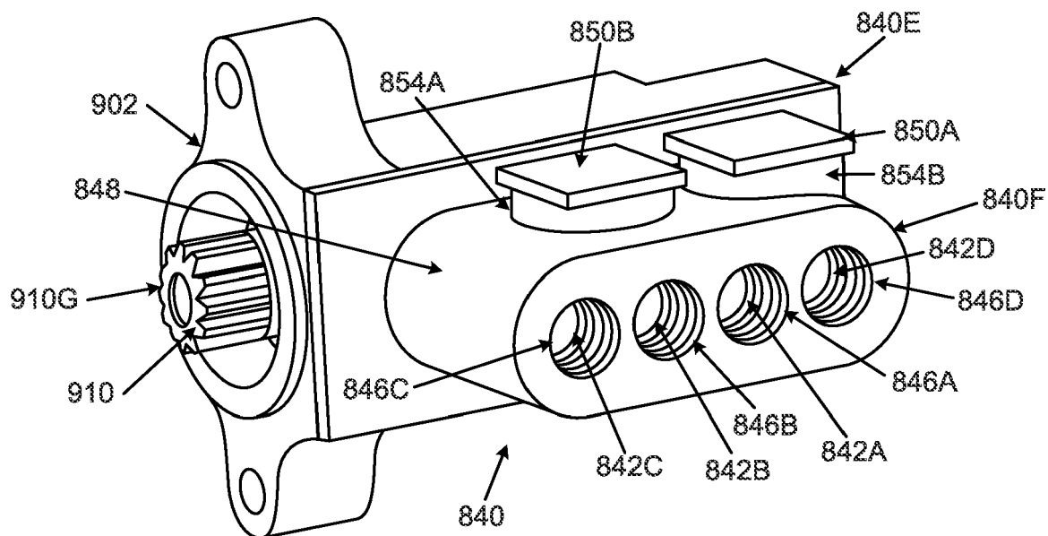
FIG. 35A
