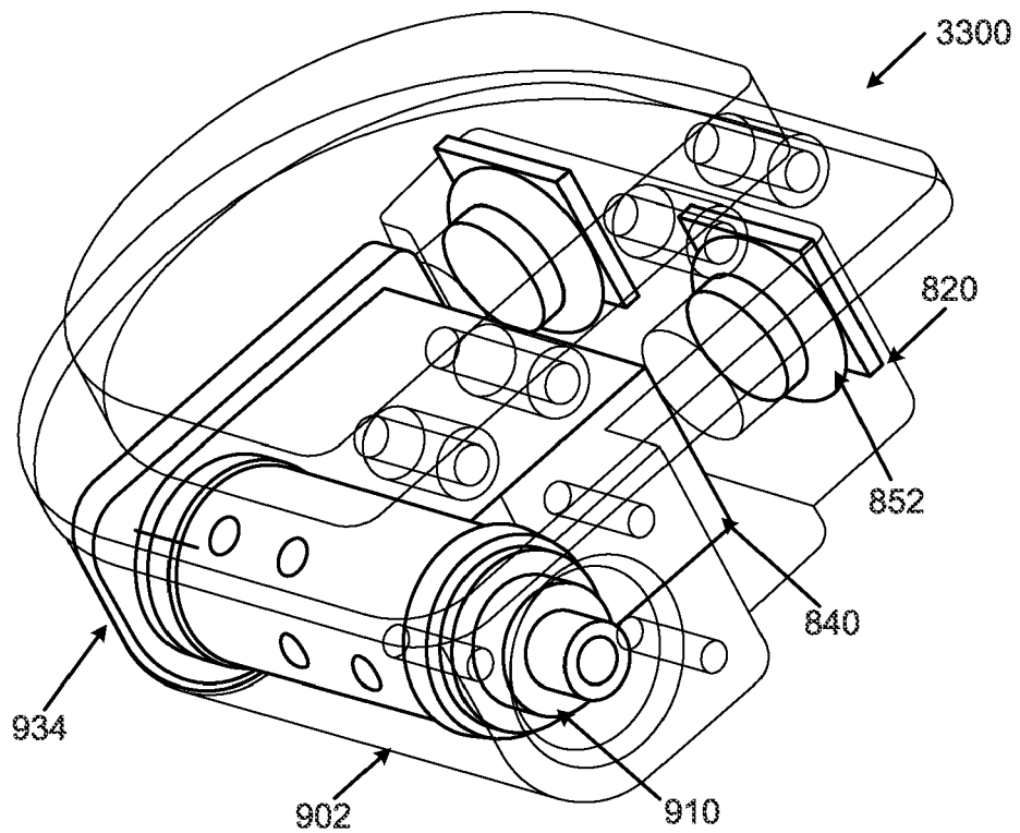
FIG. 33C
