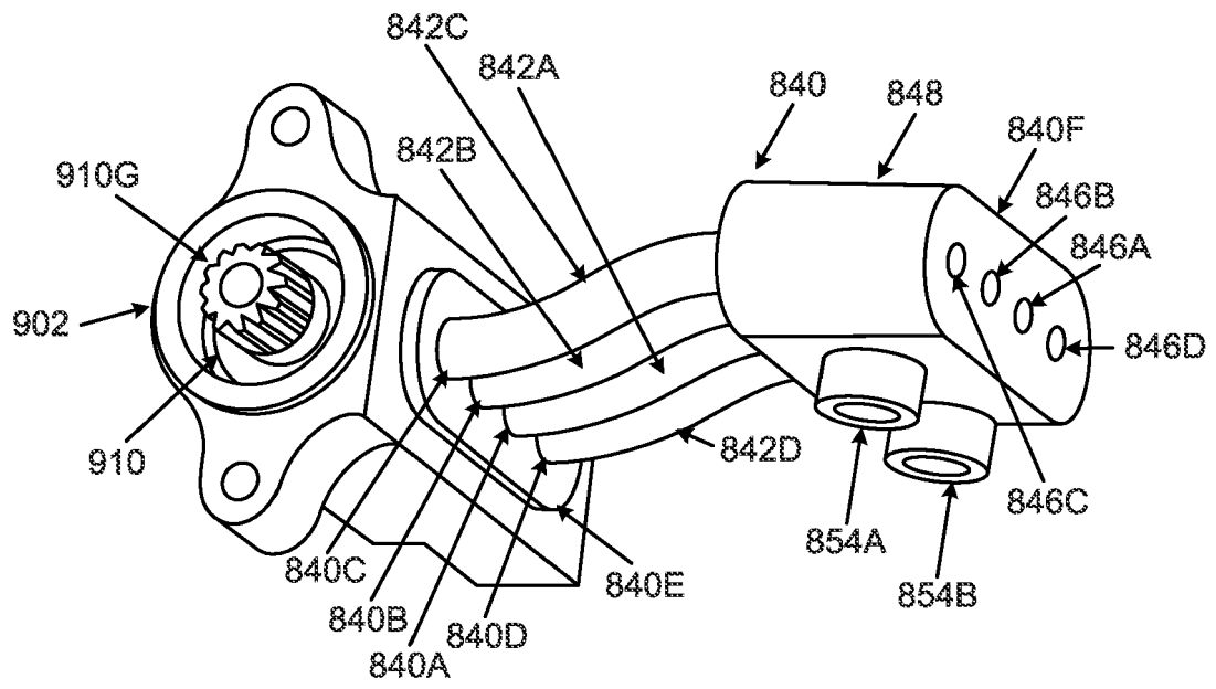
FIG. 34A
