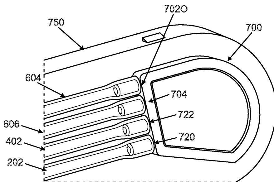
FIG. 15E
