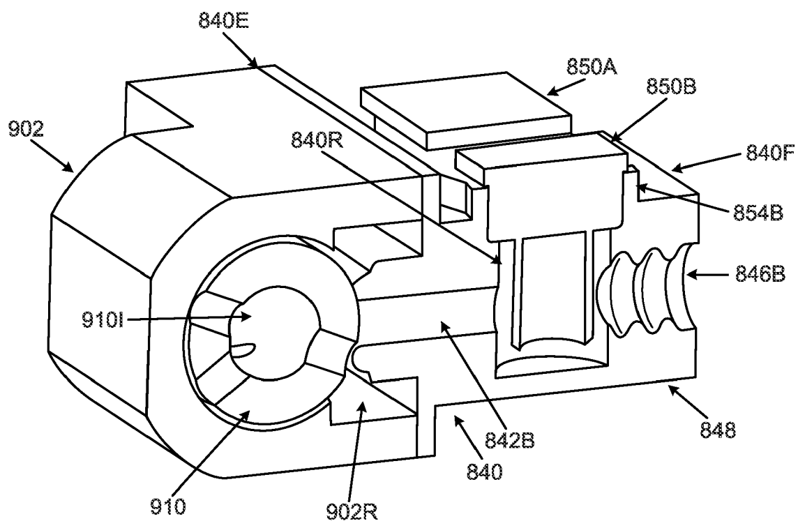
FIG. 35B
