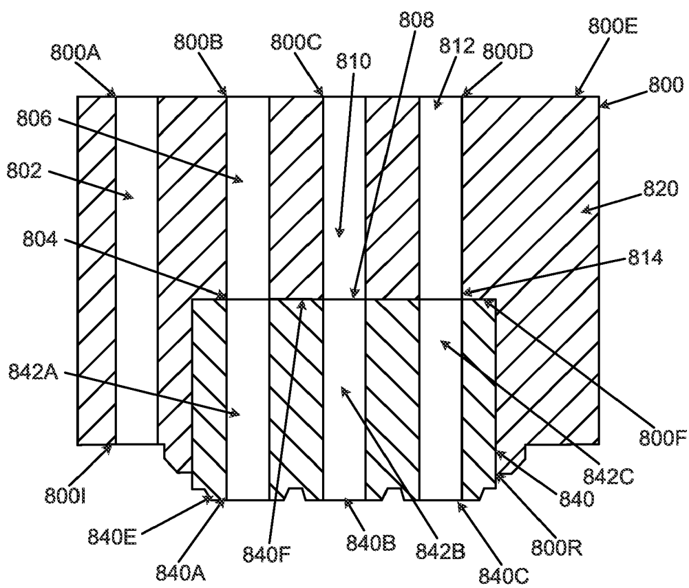
FIG. 32B
