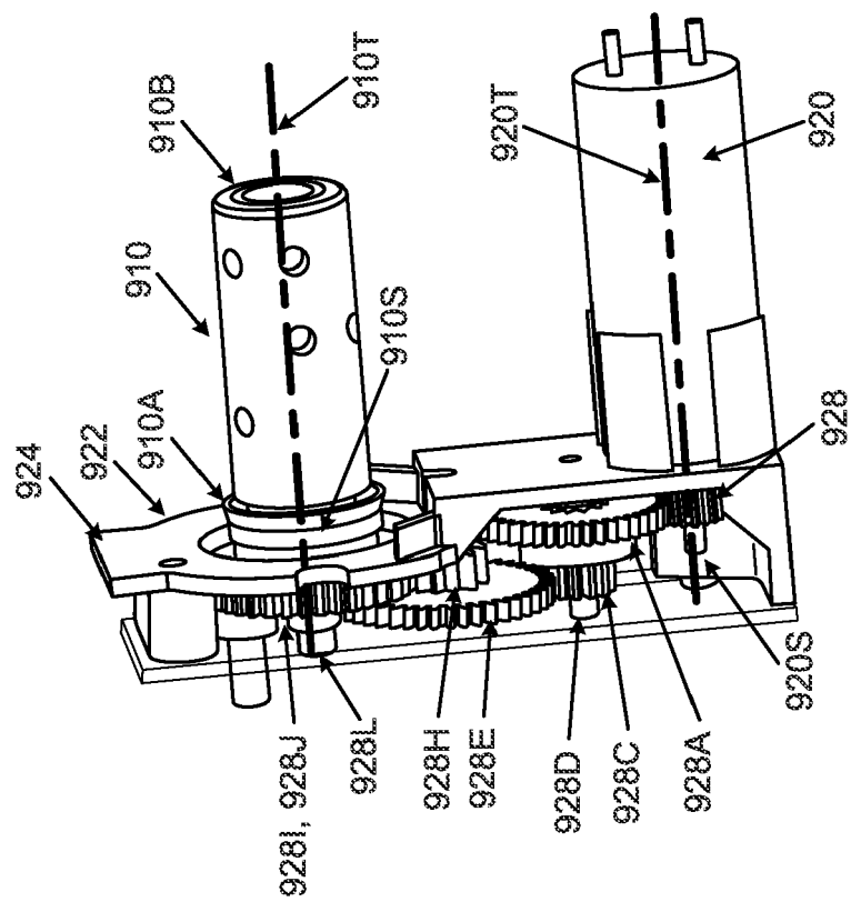
FIG. 40B
