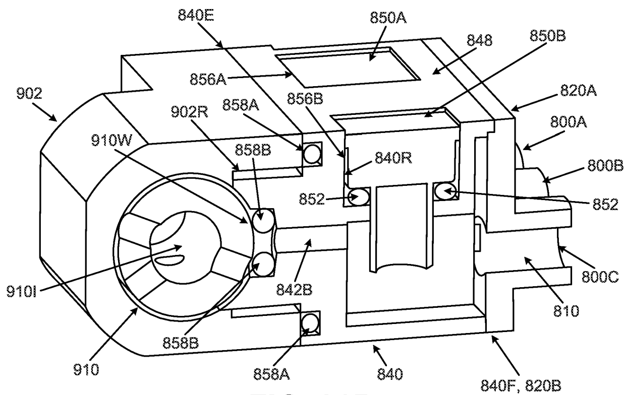
FIG. 36B
