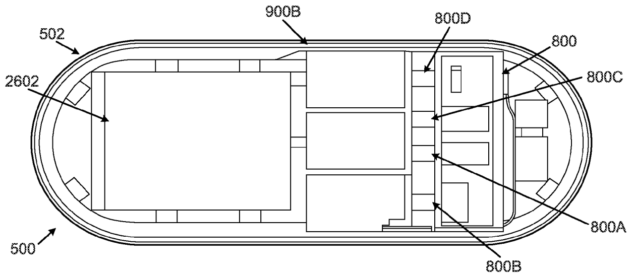
FIG. 44B
