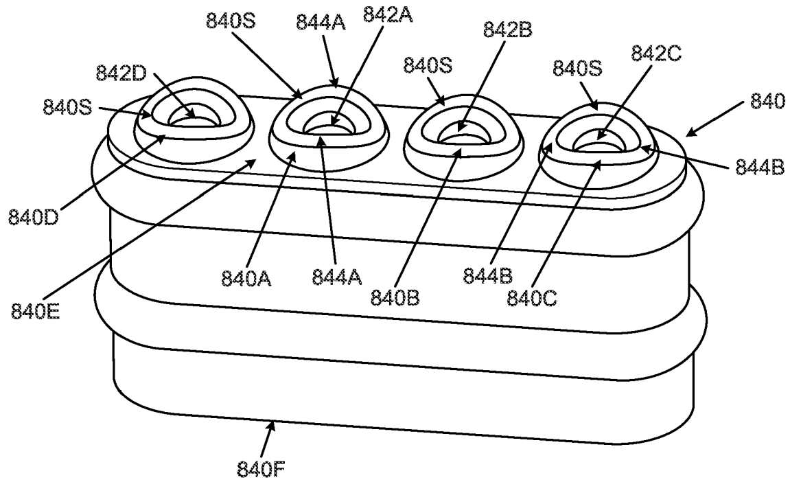
FIG. 32C
