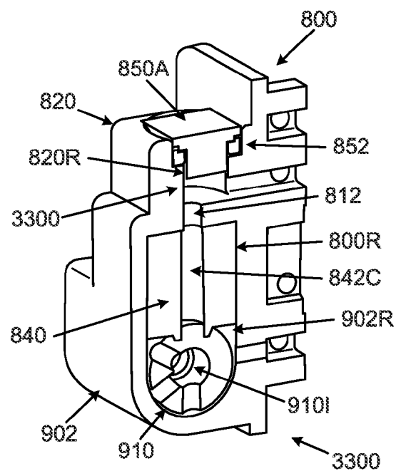
FIG. 33E
