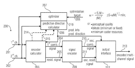
FIG 2 (AUDIO ENCODER)
