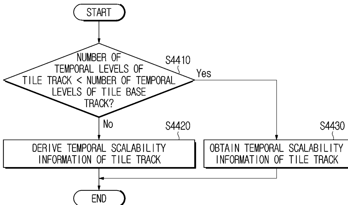
FIG. 44
