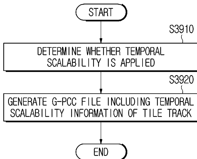
FIG. 39
