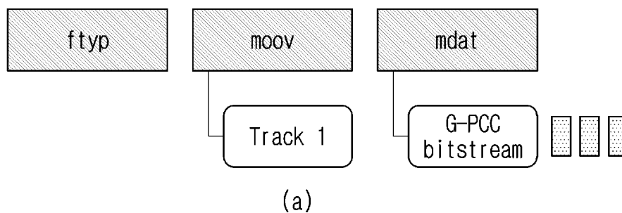
FIG. 34
