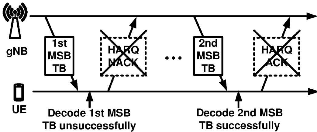
FIG. 29C
