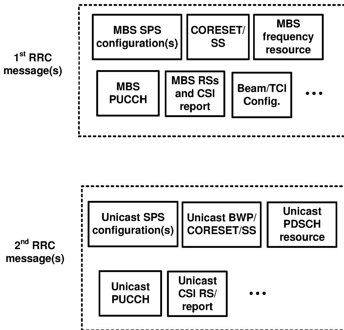
FIG. 33
