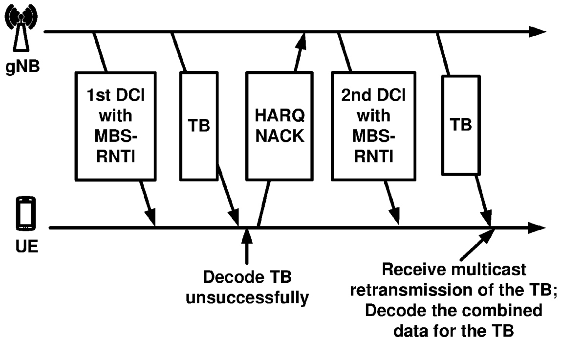
FIG. 30A
