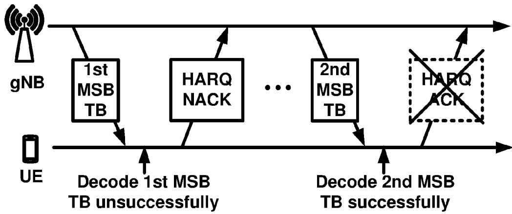
FIG. 29B
