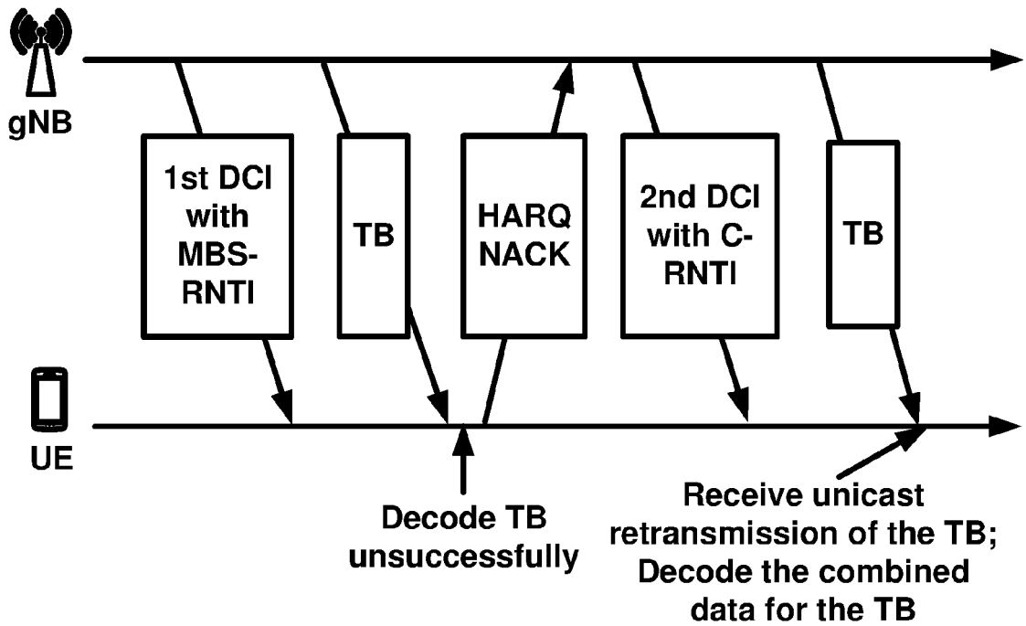
FIG. 30B
