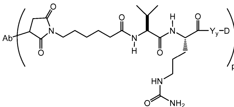
MC-val-cit
