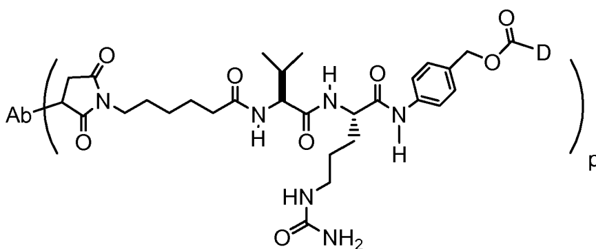
MC-val-cit-PAB
