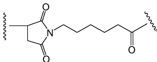
MC
