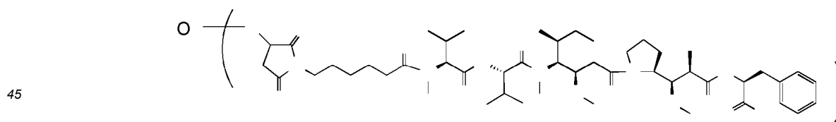
Ab-MC-MMAF (mcMMAF)
