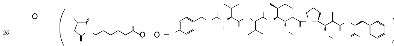
Ab-MC-vc-PAB-MMAF (vcMMAF)
