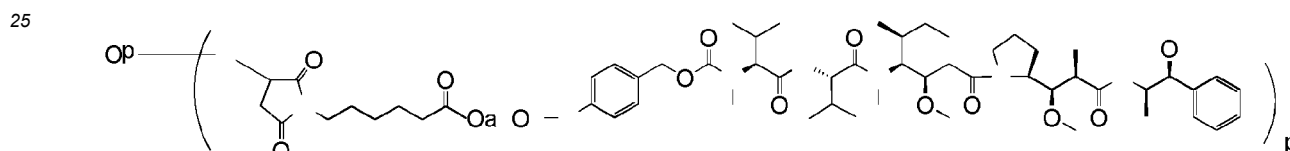
Ab-MC-vc-PAB-MMAE (vcMMAE)
