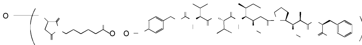
Ab-MC-vc-PAB-MMAF (vcMMAF)
