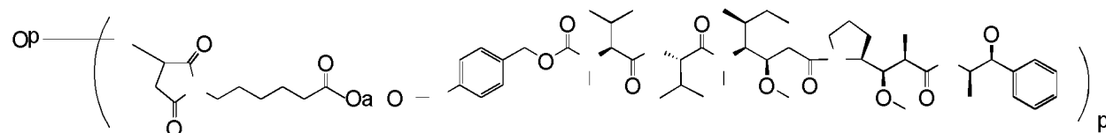
Ab-MC-vc-PAB-MMAE (vcMMAE)
