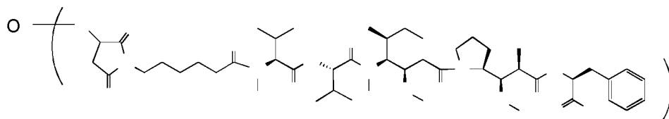
Ab-MC-MMAF (mcMMAF)
