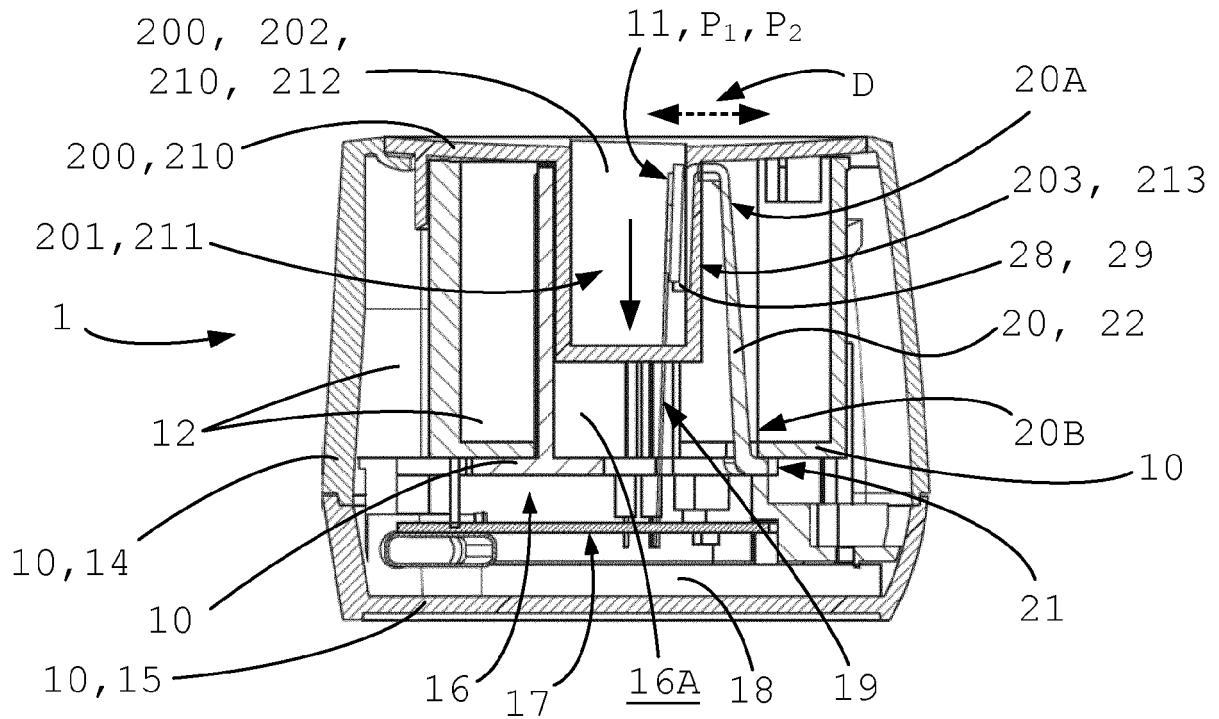
Fig 8A (A-A)
