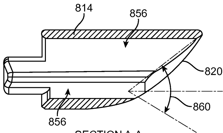
SECTION A-A FIG. 8E2
