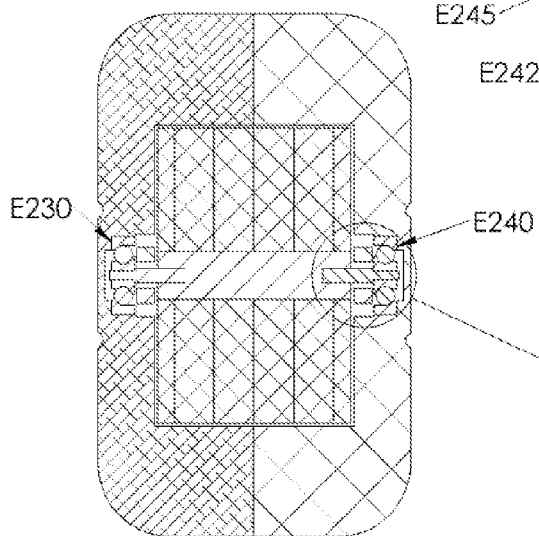
FIG. 13I SECTION D-D
