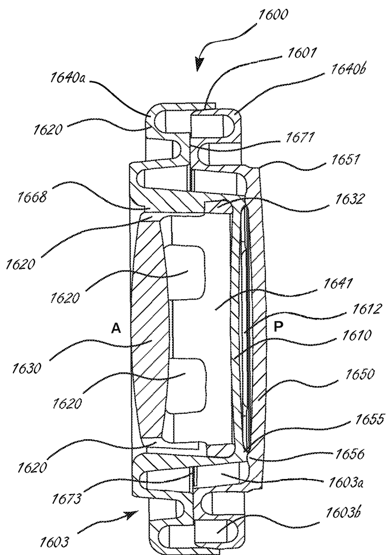
SECTION A-A
