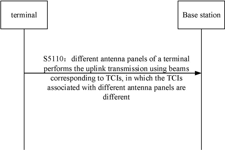
FIG. 5C
