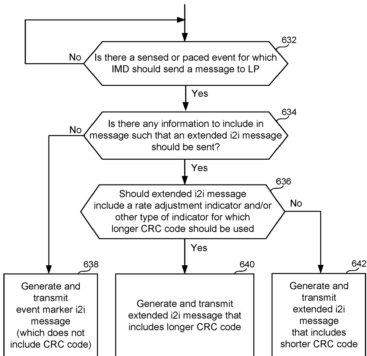
FIG. 6D
